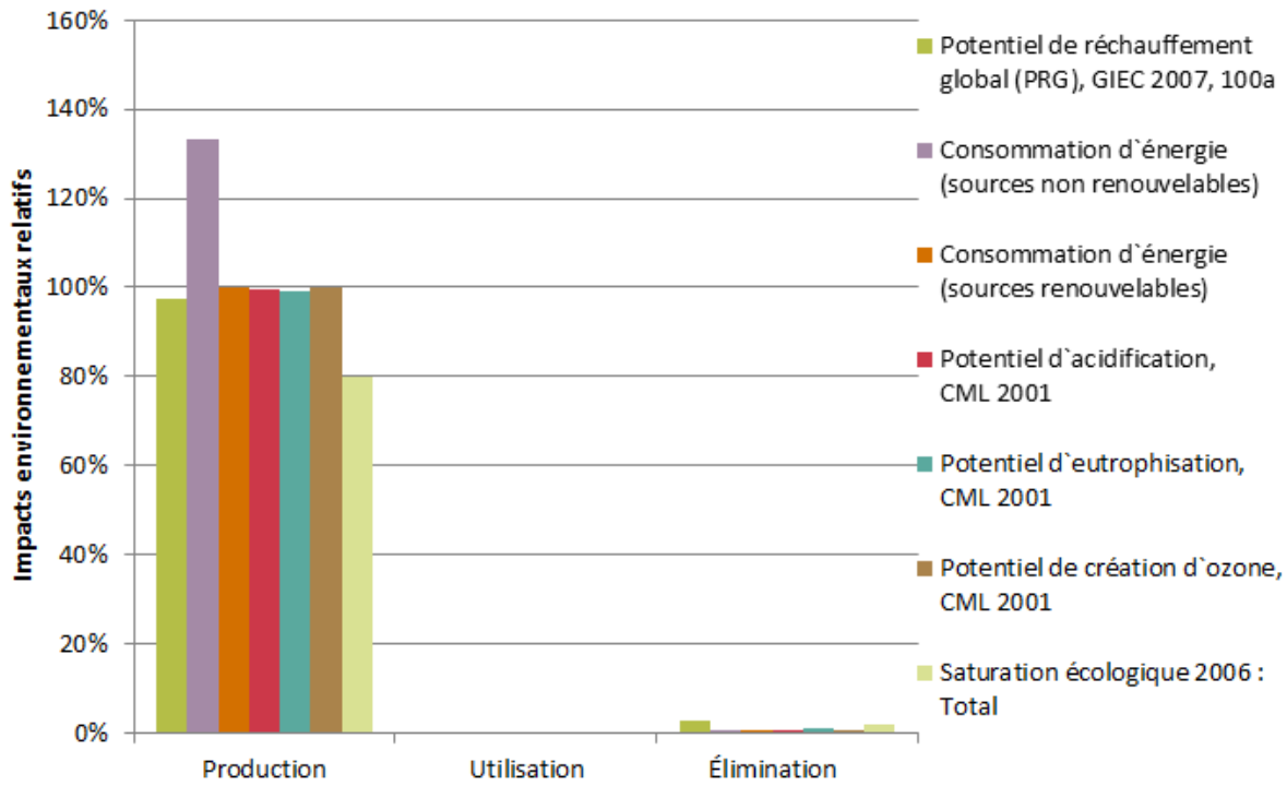
EGT346F022 (passif)
