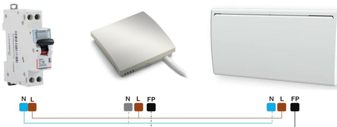
Commutateur STFP2 (fil pilote)
